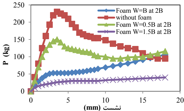
شکل ۹: فوم با عرض متغیر در عمق 2B از کف پی
