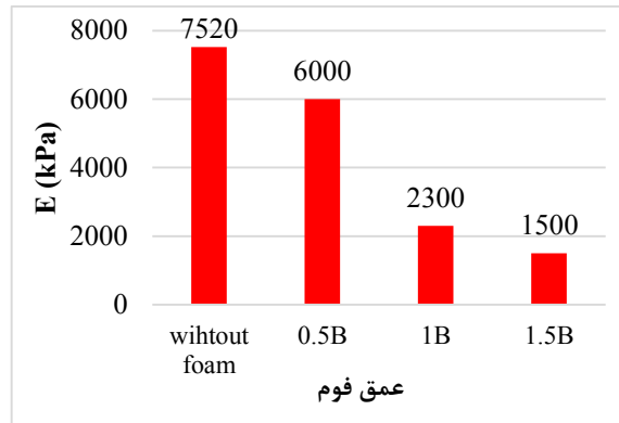
شکل ۱۰: سختی بستر ماسه ای با وجود فوم با عرض متغیر در عمق 2B از کف پی
