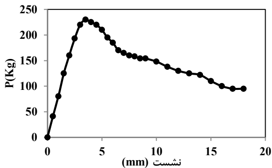
شکل ۶: منحنی بار-نشست پی مدل نواری
