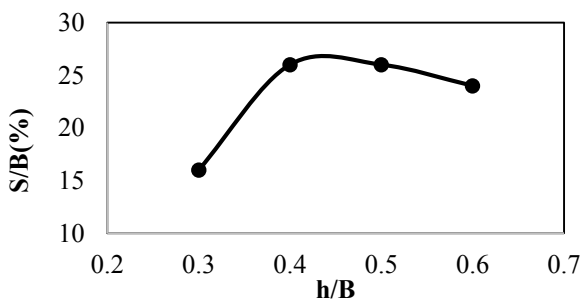
شکل ۱۹: منحنی تغییرات نسبت نشست بستر در برابر h/B های مختلف
