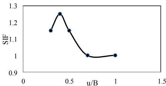
شکل ۱۲: منحنی SIF در برابر u/B
