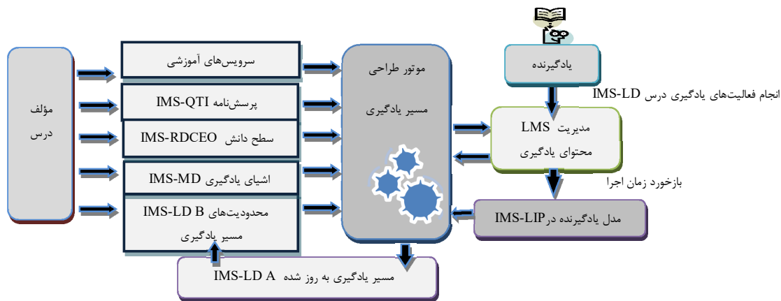
شکل ۷-معماری سيستم آموزشي
