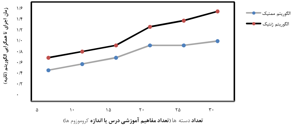
شکل ۹- مقایسه زمان اجرای الگوریتم‌های ممتیک و ژنتیک با کروموزوم‌های متفاوت
