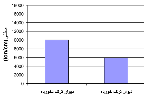
شکل ۴ اثر ترک خوردگی در سختی سازه دارای دیوار ساده و بتن با مقاومت ۳۰ مگاپاسکال
