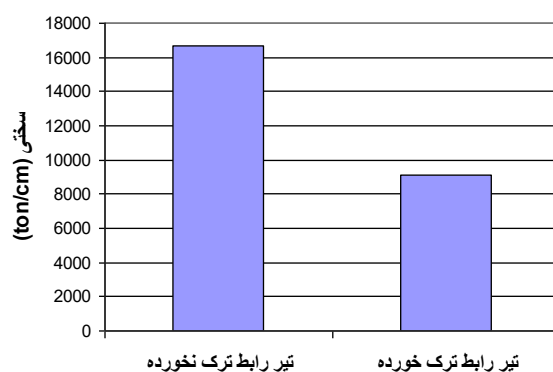
شکل ۳ اثر ترک خوردگی در سختی سازه دارای دیوار کوبله و بتن با مقاومت ۳۰ مگاپاسکال
