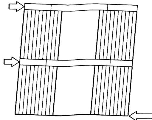
شکل ۲ نحوه عملکرد دیوارهای کوبله
