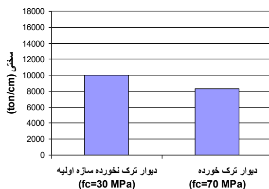
شکل ۵ اثر ترک خوردگی در سختی سازه دارای دیوار ساده و بتن با مقاومت ۷۰ مگاپاسکال
