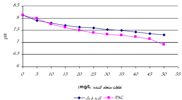
نمودار ۱ مقایسه افت PH در حذف کدورت با کلرید فریک و PAC
