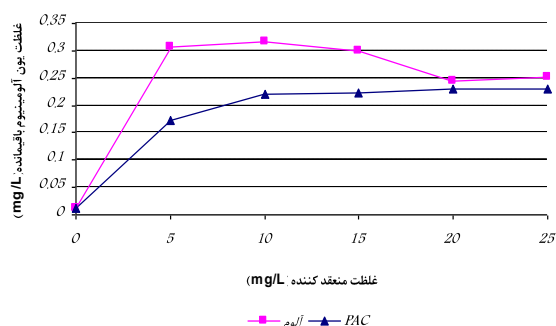
نمودار ۴ مقایسه غلظت باقیمانده یون آلومینیوم پس از مصرف آلوم و PACI
