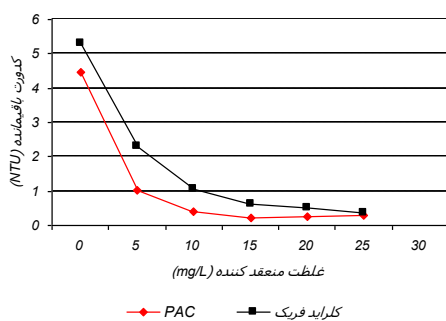
نمودار ۳ مقایسه قدرت حذف کدورت کلرید فریک و PACI به همراه بنتونیت
