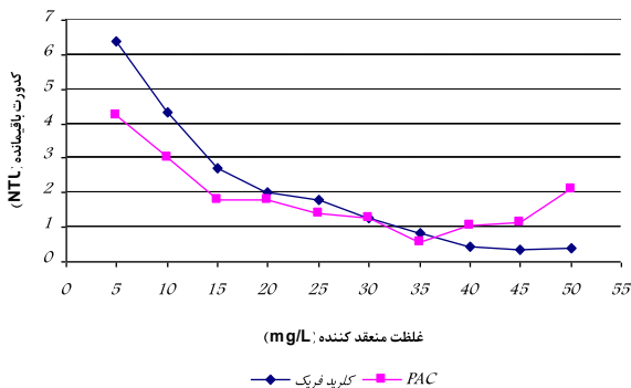
نمودار ۲ مقایسه قدرت حذف کدورت کلرید فریک و PAC
