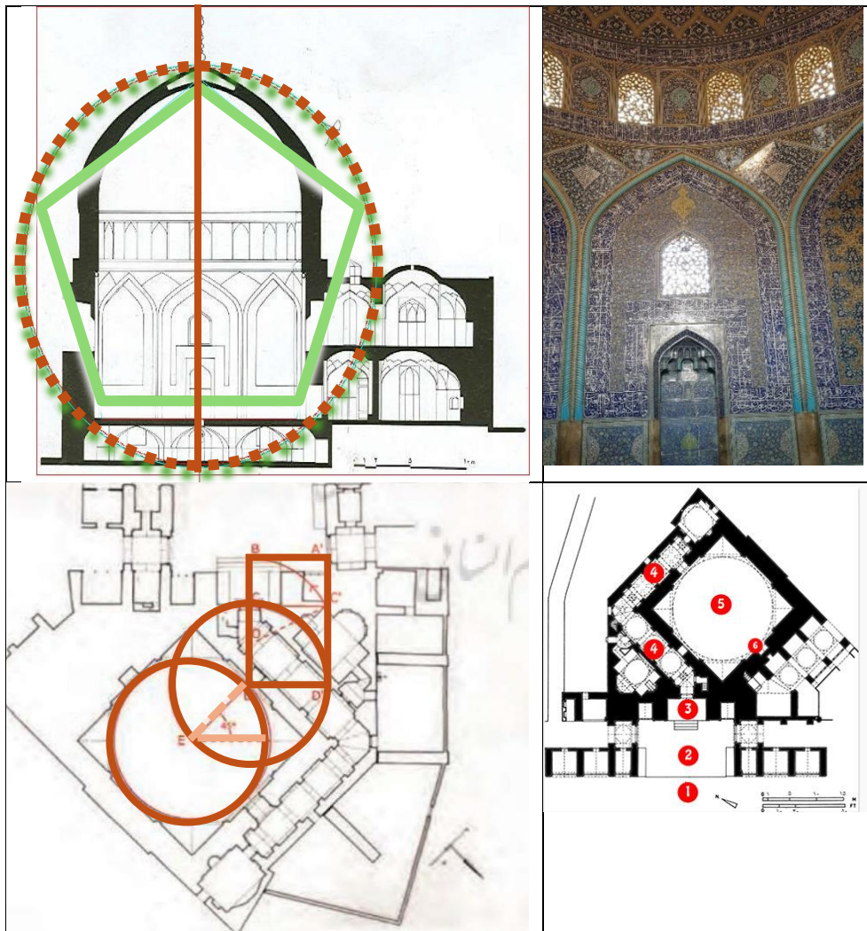
تصویر ۱۶: حرکت افقی سلسله مراتبی از ورودی تا محراب. در کنار نقش دایره در نظام هندسی مسجد شیخ لطف‌الله. ماخذ: ازدهار و همکاران، ۱۳۹۲. ترسیم دوایر مقطع از نگارنده. برخی عوامل وحدت‌بخش در معماری مسجد شیخ لطف‌الله موارد ذیل می‌باشد:
