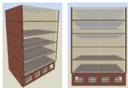
شکل 2- نمای دو پوسته دالانی
