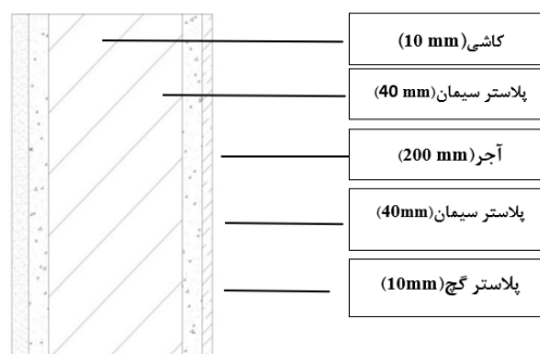
شکل ۶- لایه بندی دیوار داخلی Fig.6- Inner wall layering
