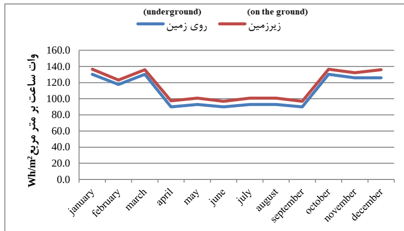
شکل 10- مقایسه مصرف انرژی روشنایی در رو و زیر سطح زمین
