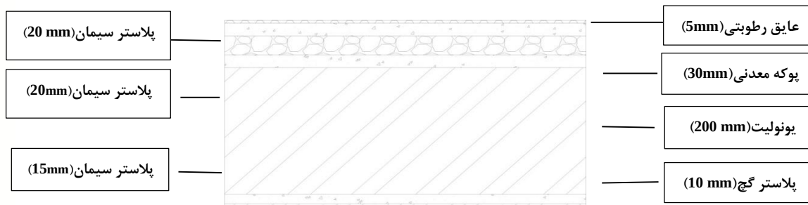
شکل ۸- لایه بندی سقف Fig.8- Roof layering
