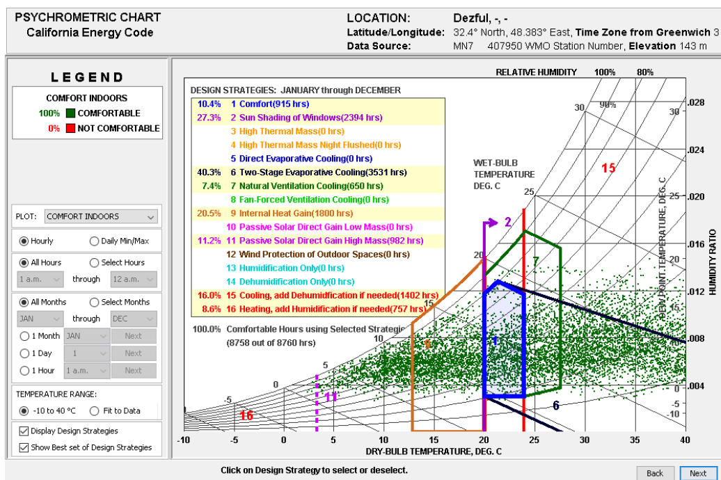
شکل ۲- استراتژی‌های طراحی در نمودار سایکرومتریک (نرم افزار ClimateConsultant)
