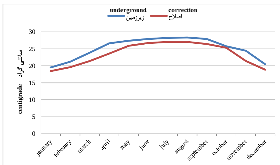
شکل 23- مقایسه دما هوا داخل ساختمان در رو و زیر سطح زمین در حالت اصلاح شده
