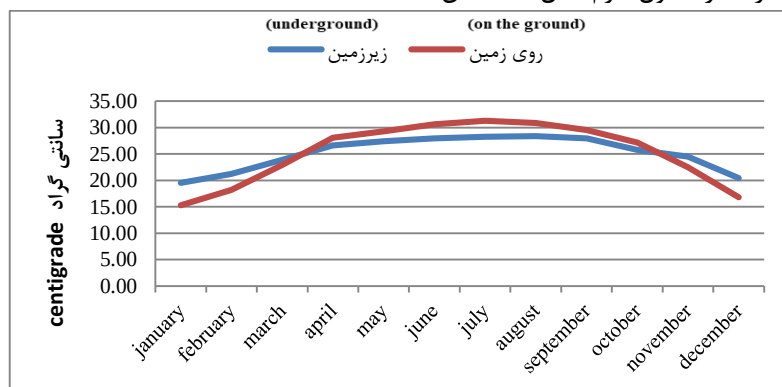
شکل 11- مقایسه دما هوا داخل ساختمان در رو و زیر سطح زمین
