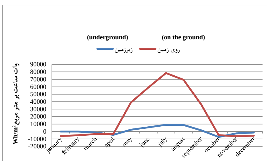
شکل 9- مقایسه اتلاف حرارت از طریق تهویه در رو و زیر سطح زمین
